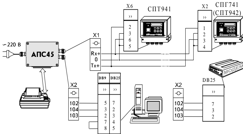
Рисунок 1 Схема подключения адаптера
